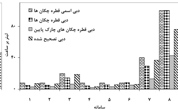
شکل ۱- الف، نمودار دبی قطره‌چکان‌ها (راست) و شکل ۱- ب، نمودار حجم آب روزانه درختان (چپ).
