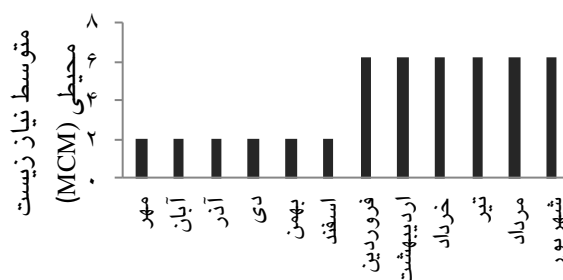
شکل ۸- تقاضای آب زیست محیطی پایین دست سد مهاباد.
