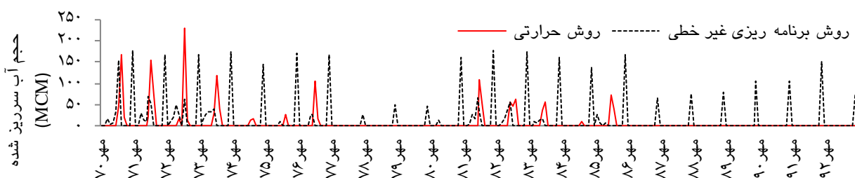
شکل ۱۳- حجم آب سرریز شده حاصل از روش‌های برنامه‌ریزی غیر خطی و روش حرارتی.
