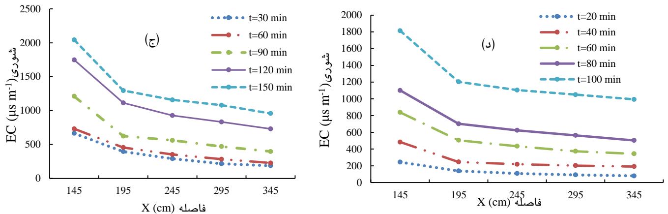
شکل ۳- نمودار زمان، شوری و فاصله به ترتیب در سرعت‌های باد (الف) ۰.۷، (ب) ۰.۸، (ج) ۰.۹ و (د) ۱.۰ متر بر ثانیه.
