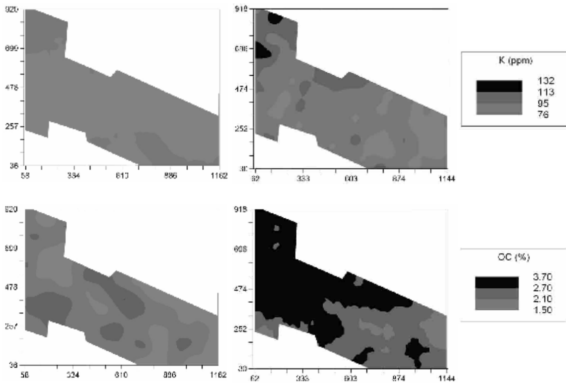
شکل 2- نقشه هم‌ارز کریجینگ متغیرها در قبل و بعد از تسطیح
