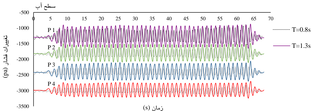
شکل ۵- سری زمانی نوسانات فشار دینامیک موج ثبت شده توسط مبدل‌های فشار در تخلخل ۱۶ درصد.
