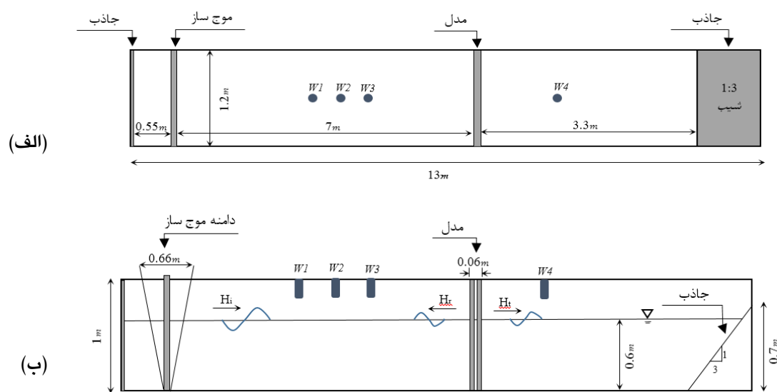
شکل ۲- کانال آزمایشگاهی. (الف): دید از بالا - (ب): دید از مقابل.
