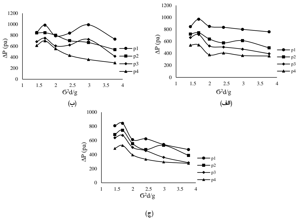
شکل ۶- تغییرات و توزیع فشار موج منظم وارد بر سازه موج شکن نفوذپذیر در H/d = 0.1 . (الف) تخلخل ۱۶ درصد. (ب) تخلخل ۱۹ درصد. (ج) تخلخل ۲۳ درصد.
