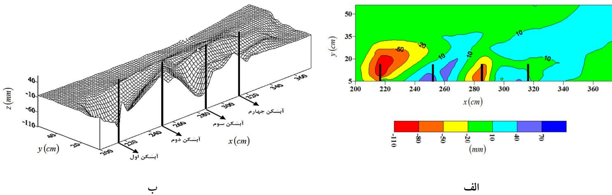
شکل ۹- خطوط هم‌تراز بستر (الف) و نمای سه‌بعدی تغییرات بستر (ب) اطراف سری آبشکن‌های صلب Fr = 0.24 ، (\alpha = 0) .
