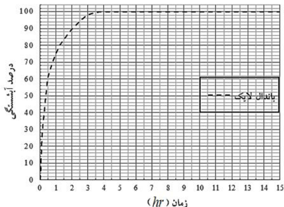
شکل ۲- گسترش آبشستگی با زمان در آزمایش تعادل.
