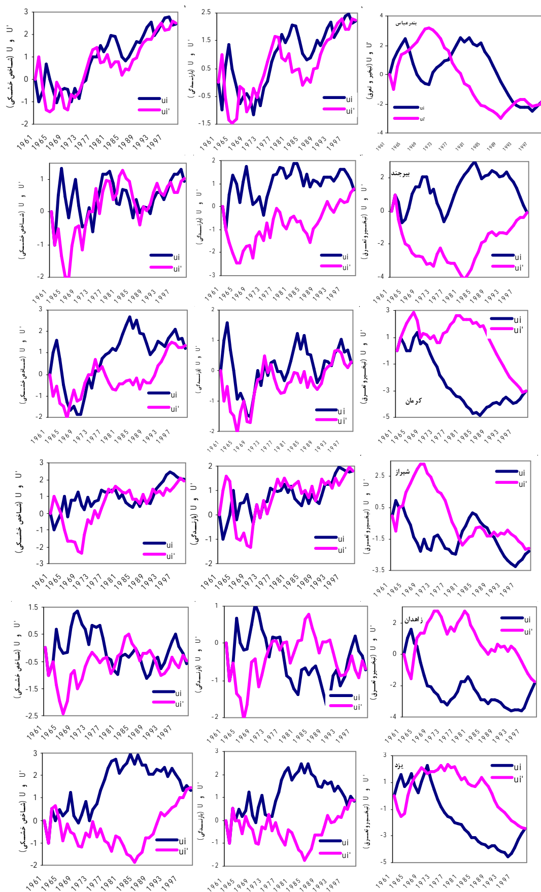
شکل 2- نمودار من کندال برای بارندگی، تبخیر و تعرق و شاخص خشکی در دوره آماری مورد مطالعه
