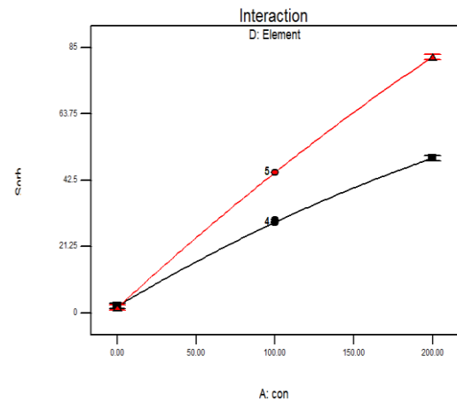
شکل ۲- جذب مس و کادمیم از محلول آبی به وسیله کیتوزان در pH برابر ۴/۵ و قدرت یونی برابر ۰/۰۳ مولار.
