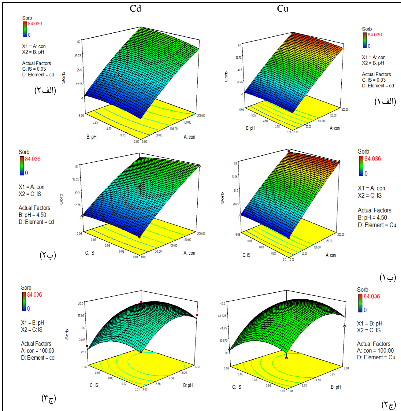
شکل ۱- نمودار سه بعدی جذب مس و کادمیم بوسیله کیتوزان الف: اثرات متقابل pH و غلظت (Con) در قدرت یونی ثابت ۰/۰۳ (mol L -1 ) ب: اثرات متقابل قدرت یونی (IS) و غلظت (Con) در pH برابر ۴/۵ ج: اثرات متقابل pH و قدرت یونی (IS) در غلظت ثابت ۱۰۰ (mg L -1 ).
