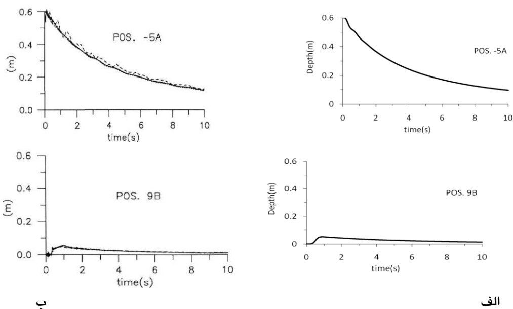
شکل ۹- هیدروگراف رقوم سطح آب در نقاط مختلف الف) محاسبه شده توسط مدل حاضر ب) اندازه گیری شده با ارتفاع سنج (خط نقطه) و گیج فشار (خط ممتد) و محاسبه شده (خط چین) توسط (فراکارولو و تورو ۱۹۹۵).
