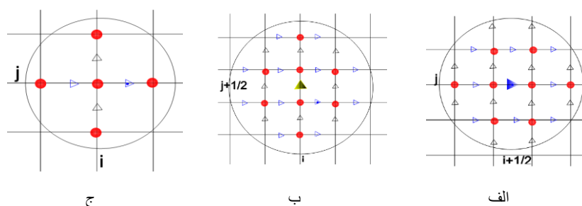
شکل ۱- الف) گره‌ای که U مومنتم بر آن منفصل می‌شود ب) گره‌ای که V مومنتم بر آن منفصل می‌شود ج) گره‌ای که پیوستگی \eta بر آن منفصل می‌شود.
