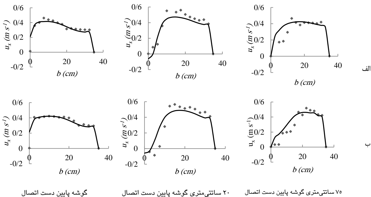
شکل ۵- مقایسه پروفیل‌های عرضی سرعت طولی در مقاطع مختلف کانال اصلی الف) 1/5 سانتی متری از کف ب) 16/5 سانتی متری از کف (نقاط توپر اندازه گیری، خط ممتد محاسباتی با مدل).
