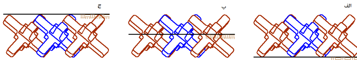
شکل ۷- رقوم مختلف کارگذاری قطعات شش‌پایه: الف) روی بستر D_1 ، ب) عمق میانی D_3 ، ج) زیر بستر D_2 .
