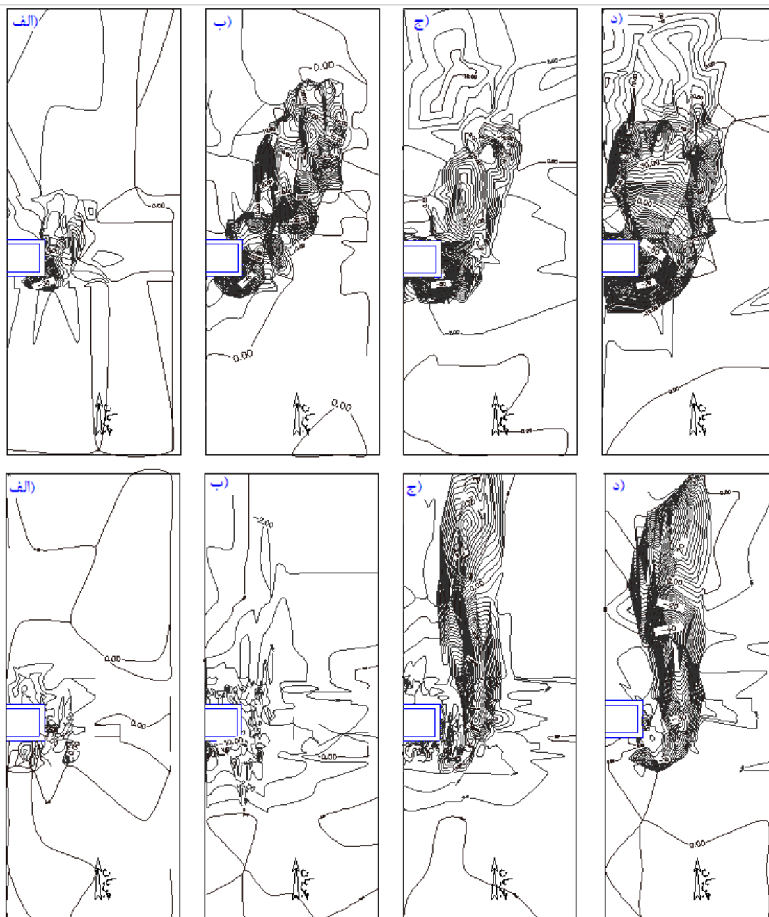
شکل ۱۱- و وضعیت کلی توپوگرافی بستر در پایان آزمایش، ردیف بالا آزمایش‌های شاهد و ردیف پایین آزمایش‌های
