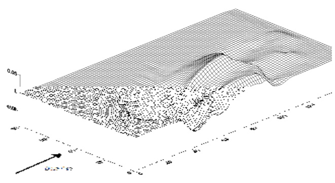
شکل 5- توپوگرافی حفره های آبستگي ایجاد شده در اطراف دو پایه پل و آبشکن.
