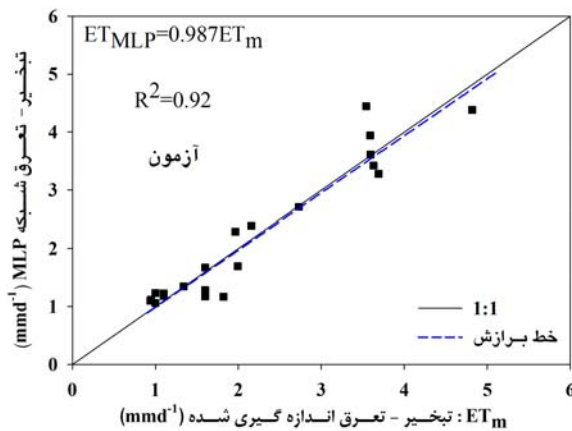
شکل ۱- مقایسه مقادیر تبخیر-تعرق مرجع اندازه‌گیری و تخمینی با شبکه MLP برای سناریو S 5 .
