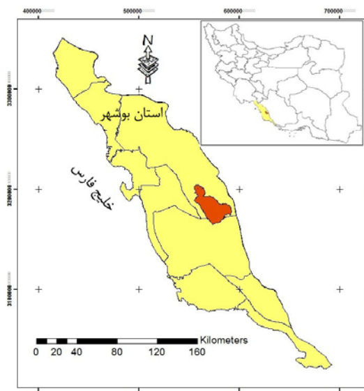
شکل ۱- موقعیت حوضه آبخیز بوشکان در استان بوشهر و کشور ایران.
