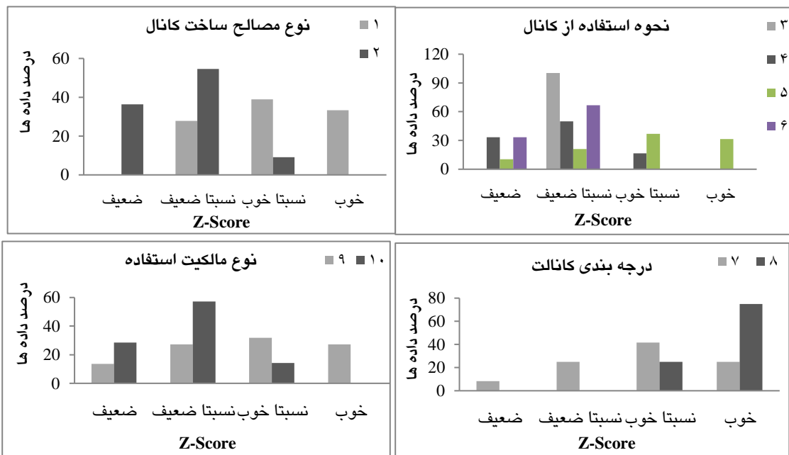
شکل ۳- میزان‌های متناسب با Z-Score محاسبه شده برای راندمان توزیع بر اساس کد بندی‌های انجام شده کانالت=۱، کانال خاکی=۲، کانالت اختصاصی=۳، کانال خاکی اختصاصی=۴، کانالت غیراختصاصی=۵، کانال خاکی غیراختصاصی=۶ کانالت درجه سه=۷، کانالت درجه چهار=۸، کانال غیراختصاصی=۹ و کانال اختصاصی=۱۰
