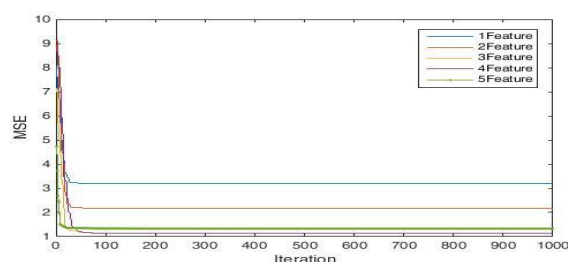
شکل ۵: نمودار همگرایی الگوریتم WCA برای ترکیب ویژگی‌های متفاوت.
