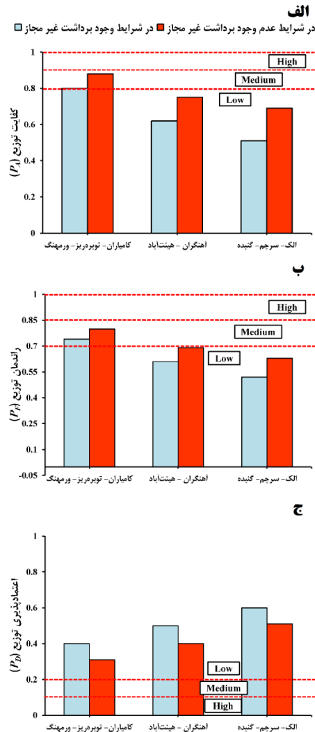
شکل ۸- نحوه تغییرات شاخص های ارزیابی مختلف، به ازای سناریوی بهره برداری چهارم (S4)، الف) شاخص کفایت توزیع (ب) شاخص راندمان توزیع (ج) شاخص اعتمادپذیری توزیع.
