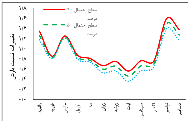
شکل ۲- مقدار تغییرات دما (راست) و بارش (چپ) در سطوح احتمالی مختلف تحت سناریوی B1.
