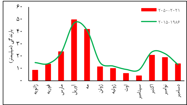
شکل ۳- مقایسه میانگین بارش ماهانه کاهش مقیاس یافته برای دوره (۲۰۲۱-۲۰۵۰) و مشاهداتی دوره پایه (۱۹۸۶-۲۰۱۵) تحت سناریوی A2 (سمت چپ) و سناریوی B1 (سمت راست).
