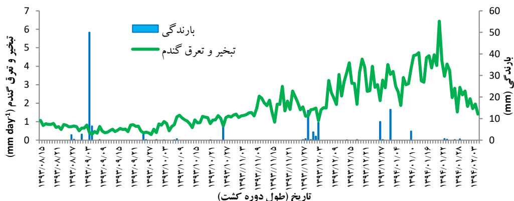
شکل ۵- نمودار تغییرات شدت تبخیر-تعرق گندم و بارندگی‌های سال زراعی ۹۳-۹۴ در منطقه مطالعاتی.
