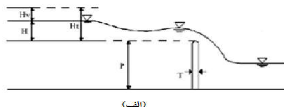
شکل ۱- پروفیل طولی سرریز کنگره‌ای، (ب) پلان سرریز کنگره‌ای.
