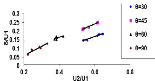
شکل ۹- مقایسه قدرت جریان ثانویه در زاویه‌های مختلف
