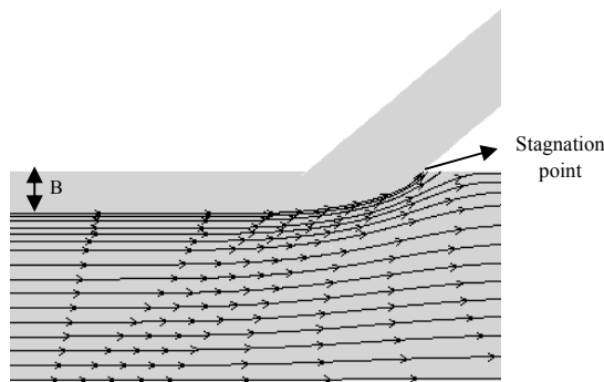
شکل ۲- عرض لوله جریان در فاصله ۱۸ سانتی‌متری از کف در عدد فرود ۰/۲۵ و نسبت آبیگری ۰/۳ در آبگیر ۳۰ درجه.
