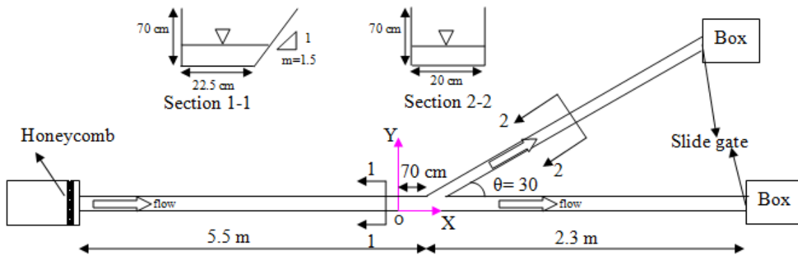
شکل ۱- پلان تجهیزات آزمایشگاهی در این مطالعه.
