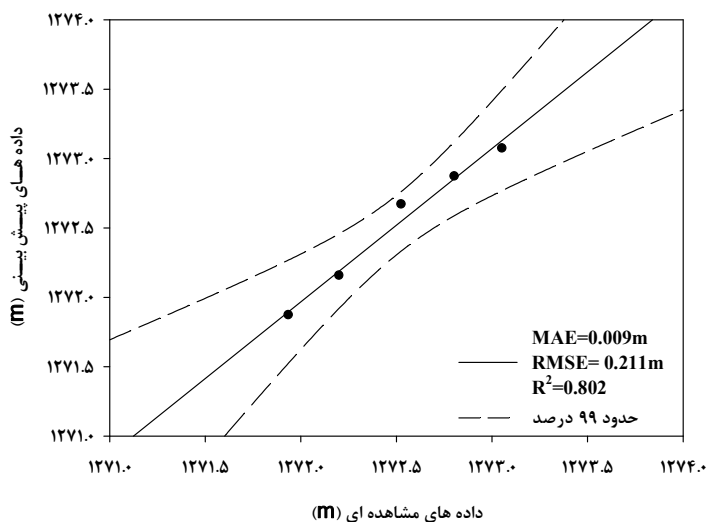
شکل ۳- نتایج بررسی و صحت سنجی مدل تلفیقی AR-ARCH در دوره آماری ۱۳۸۶-۱۳۹۰.
