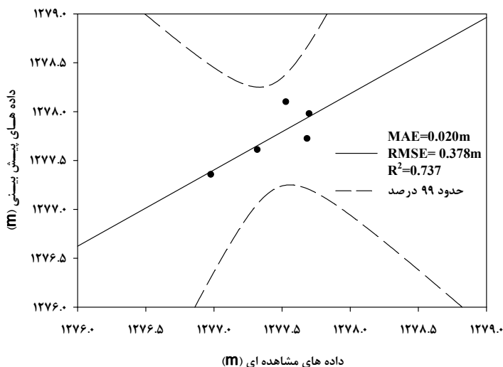
شکل ۴- نتایج بررسی و صحت سنجی مدل AR(3) در دوره آماری ۱۳۸۶-۱۳۹۰.
