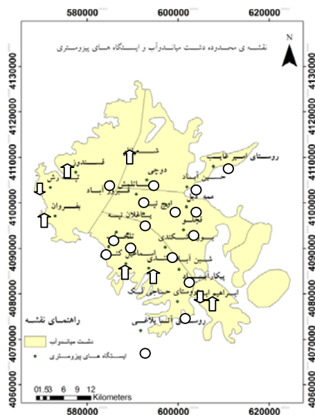
شکل ۲- نقشه روند تغییرات هدایت الکتریکی (EC) آب زیرزمینی در ماه پرب آب در دشت میاندوآب.
