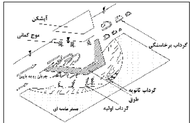
شکل 2- مکانیزم آبشستگی اطراف آبشکن با طوق
