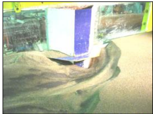
شکل 7- نمونه‌ای از حفره آبشستگی ایجاد شده در اطراف آبشکن طوق‌دار در تحقیق حاضر
