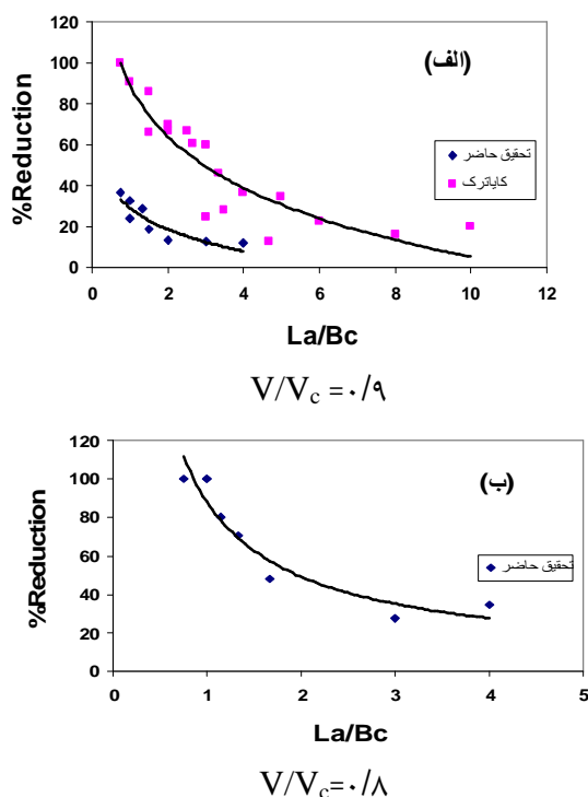
شکل 17- تاثیر \frac{L_a}{B_c} در درصد کاهش آبستگی
