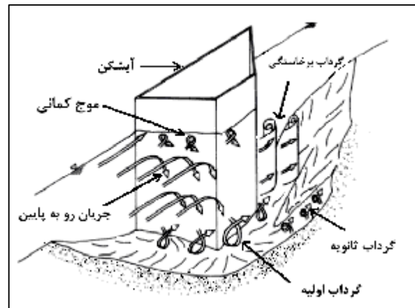
شکل 1- مکانیزم آبشستگی در اطراف آبشکن (بارهبیوا و دی 2004)
