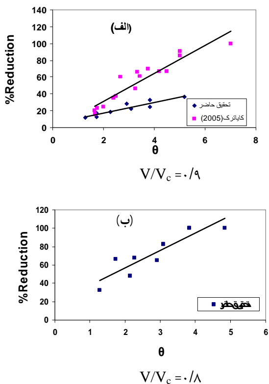
شکل 18- تاثیر پارامتر q در درصد کاهش آبستگی
