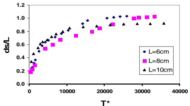
شکل 10- رابطه بین T^* و \frac{d_s}{L} برای آبشکن بدون طوق
