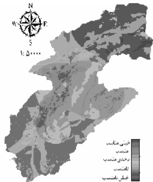
شکل 9- استعداد اراضی برای پخش سیلاب در مدل Binary evidence maps
