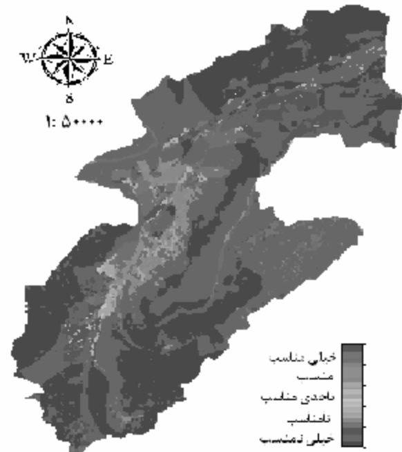
شکل 17- استعداد اراضی برای پخش سیلاب در مدل گاما 0/7
