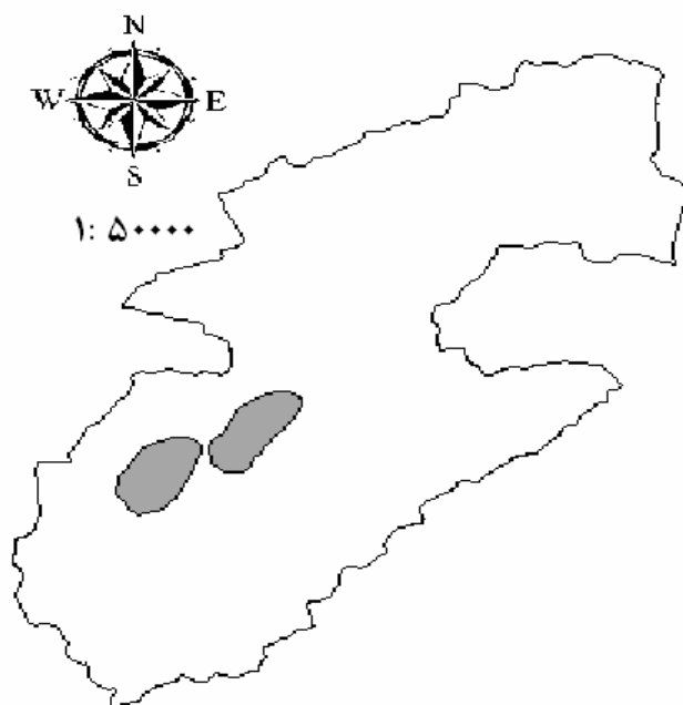
شکل 19- اراضی مستعد پخش سیلاب به روش دستی
