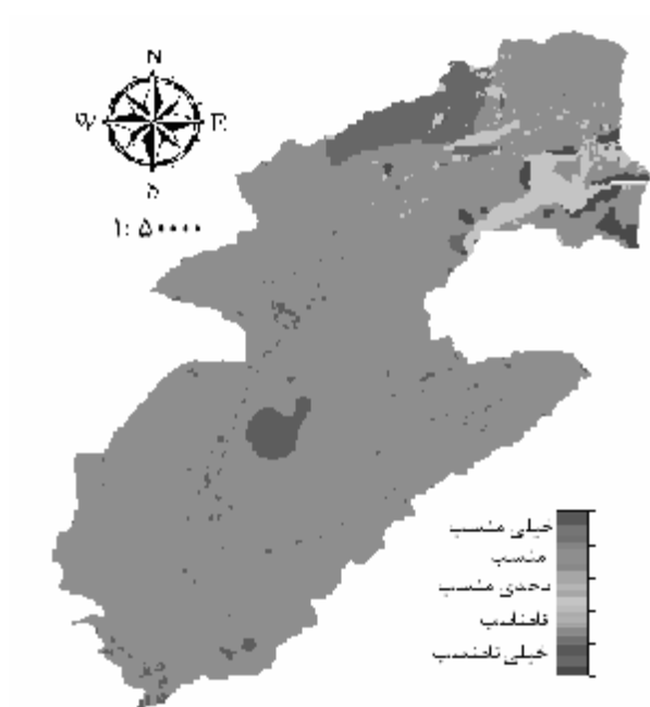
شکل 12- استعداد اراضی برای پخش سیلاب در مدل منطق فازی OR
